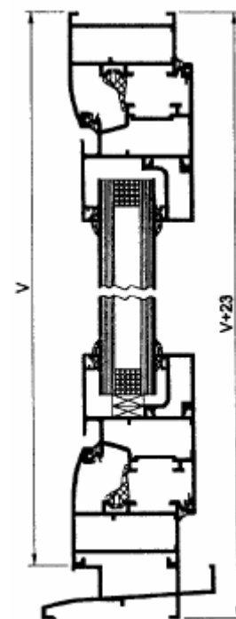
Sección B-B
