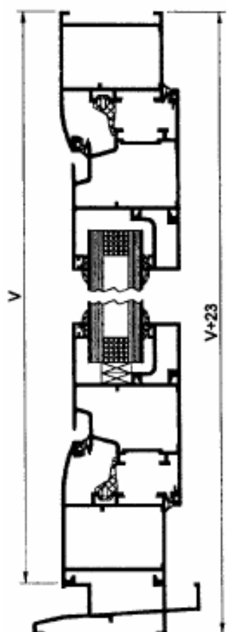
Sección B-B
