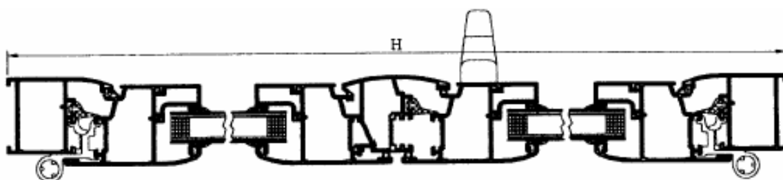
Sección A-A
