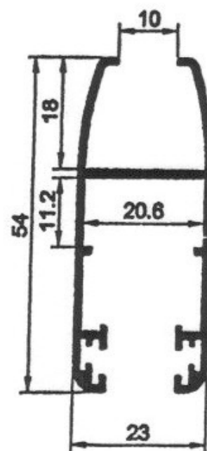
Perfil Hoja 2716
