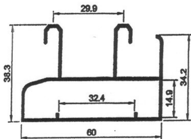
Perfil marco 2701
