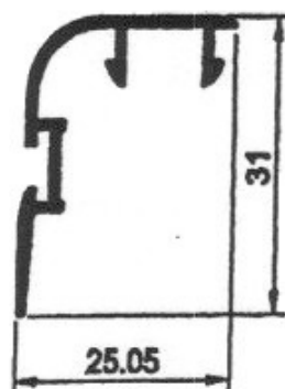
Perfil cruce 2719
