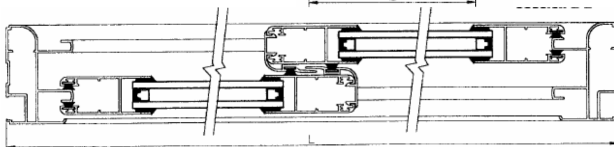
Sección A-A
