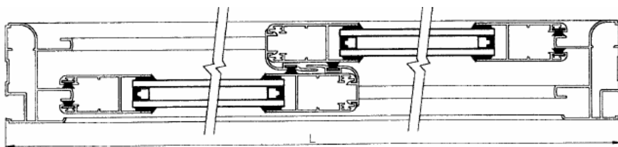
Sección A-A
