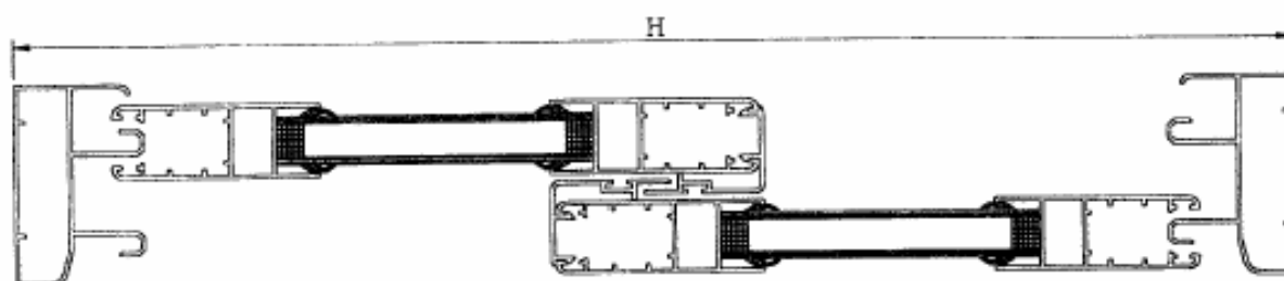
Sección A-A
