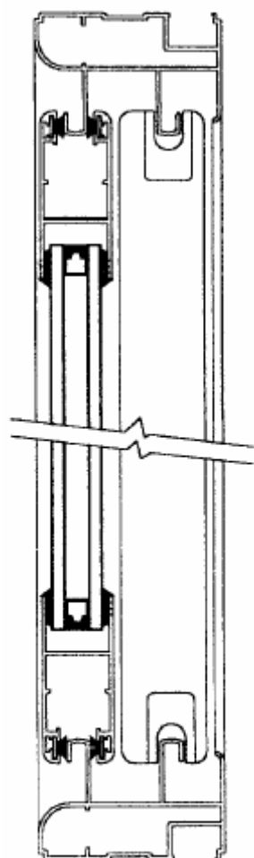
Sección B-B
