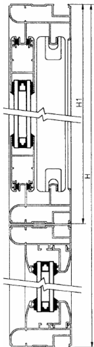
Sección B-B
